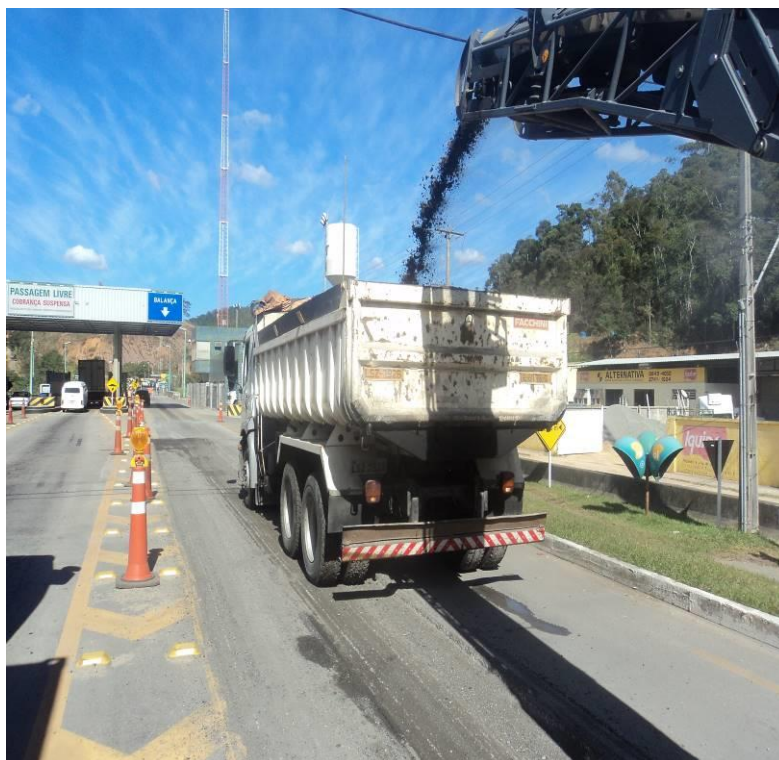
Reconstrução do Pavimento – Km 70,9 – P1 – Execução da Fresagem
